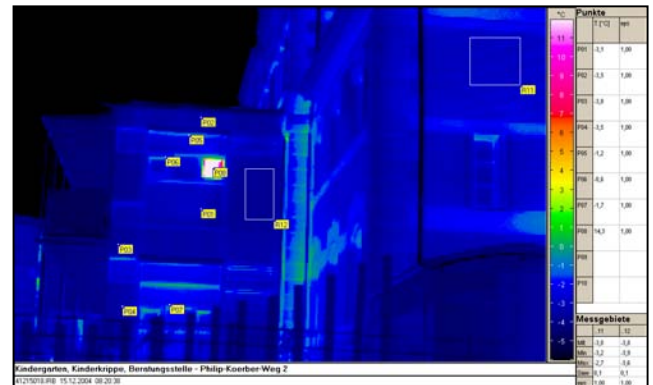
Bild 12: Wärmebild der Ostfassade Alt- und Anbau nach Sanierung
