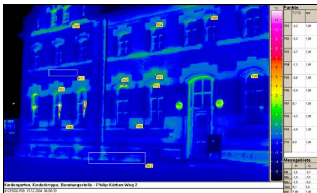
Bild 11: Wärmebild der Nordfassade Altbau nach Sanierung
